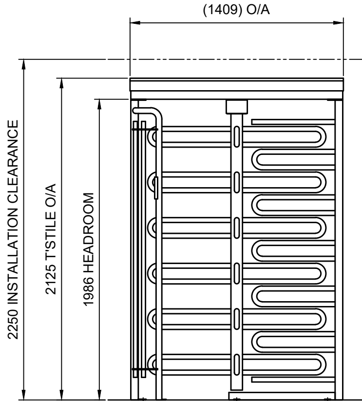
ELEVATION
