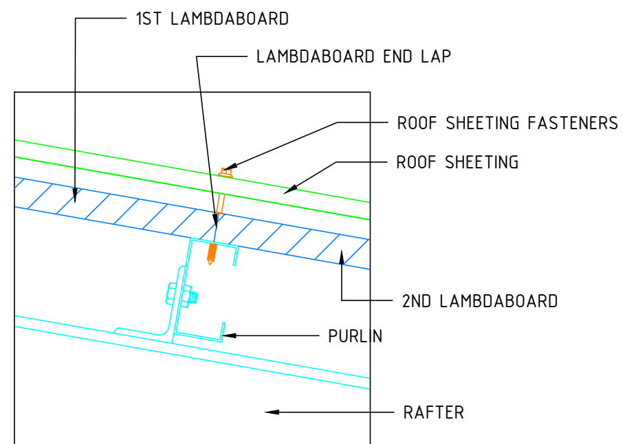
DETAIL 1 N.T.S.
