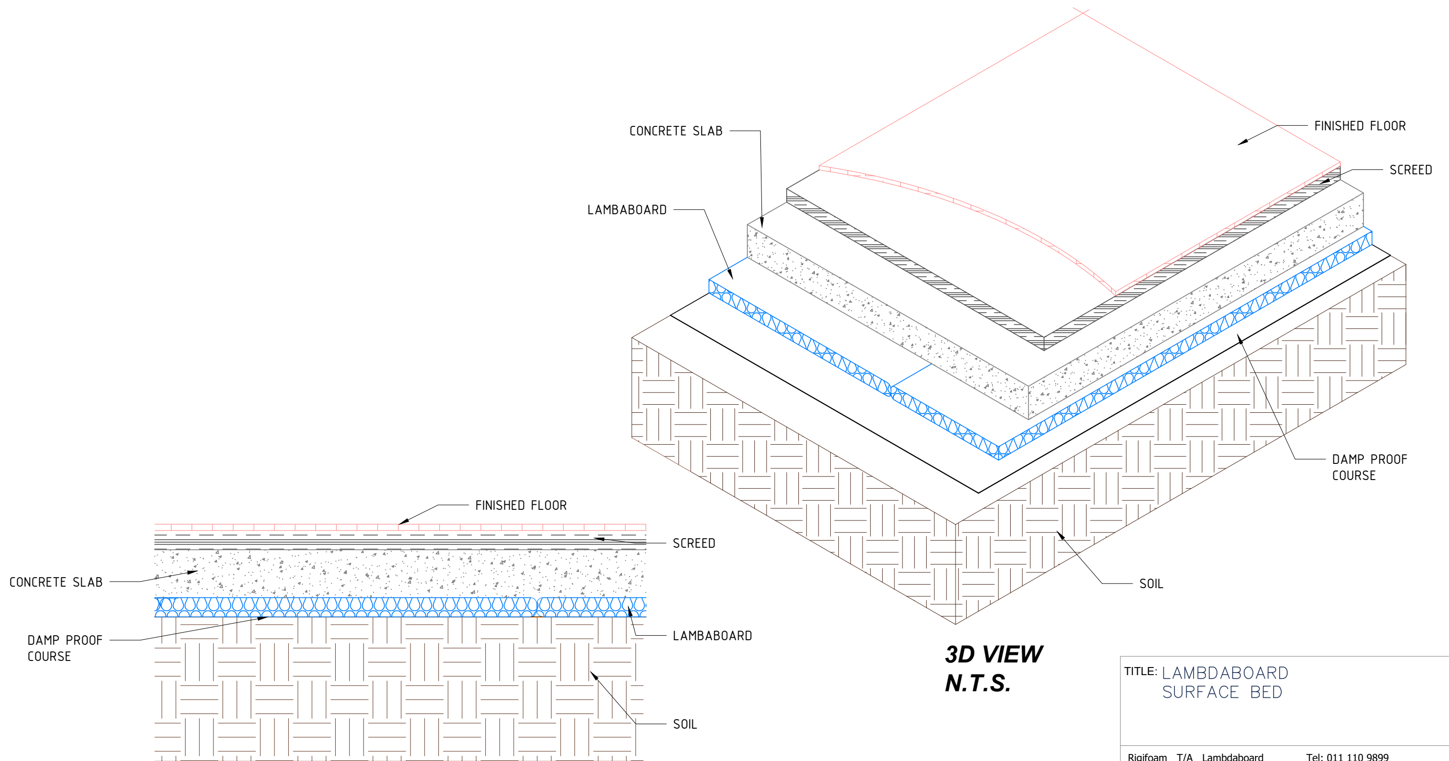
SECTION VIEW N.T.S.
