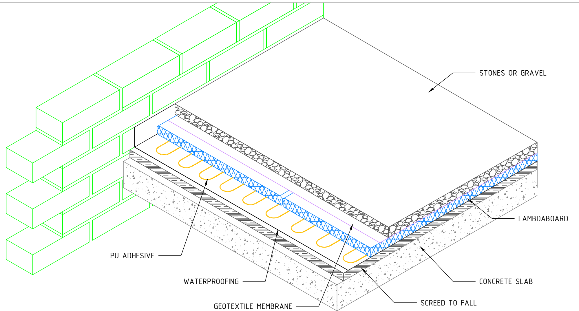
3D VIEW N.T.S.
