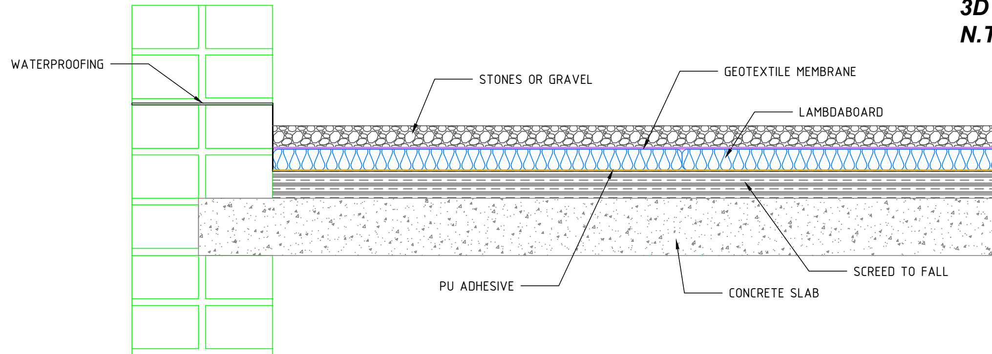
SECTION VIEW N.T.S.
