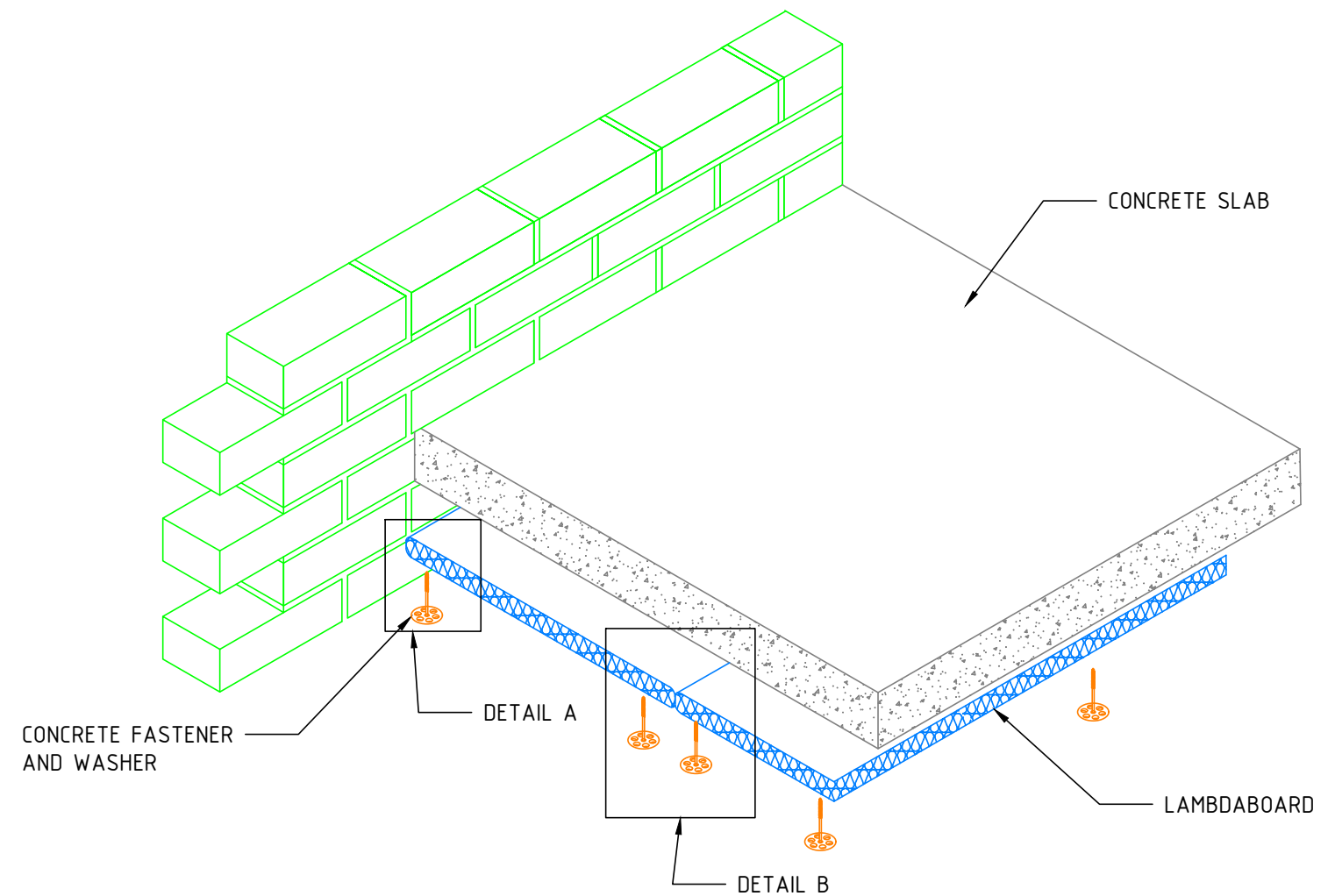
3D VIEW N.T.S.
