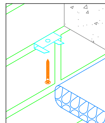
DETAIL A N.T.S.
