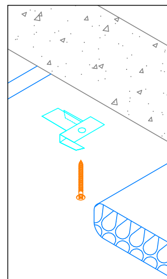
DETAIL B N.T.S.
