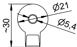
Befestigungshaken / Mounting Hook
